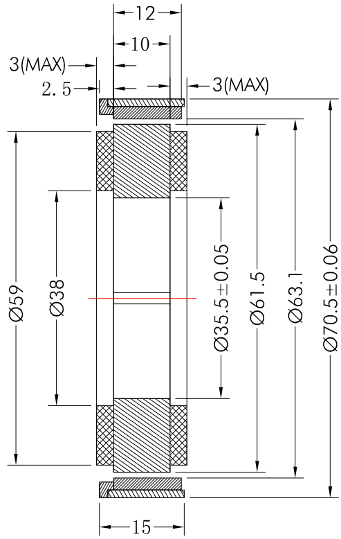
截面 A-A
