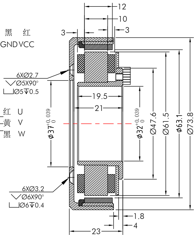
截面 A-A
